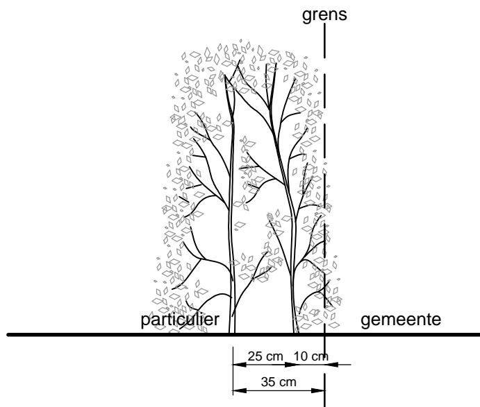
Dwarsprofiel zonder greppel
